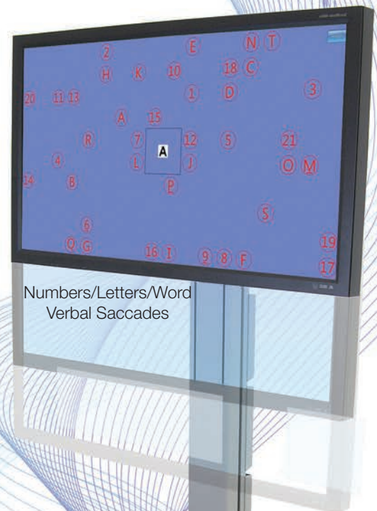
Selectable Parameters
